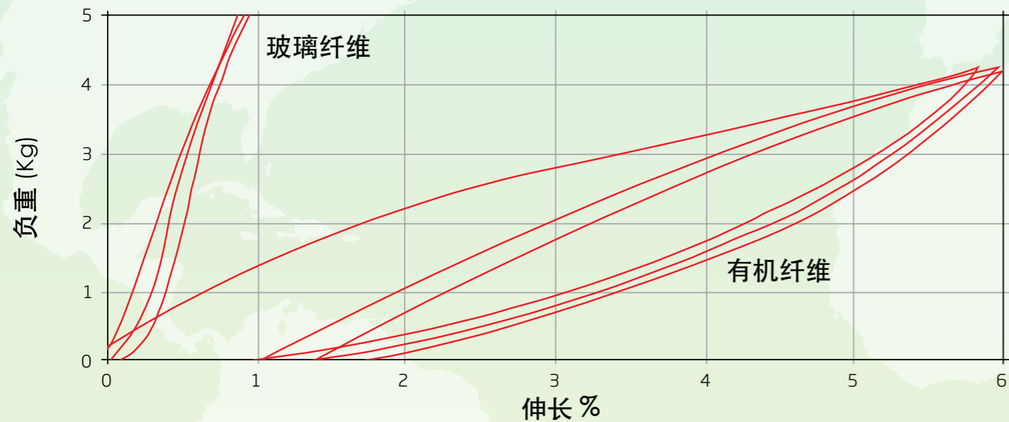
滞后曲线
